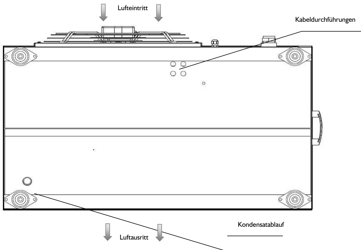
Abb.: Untersicht
