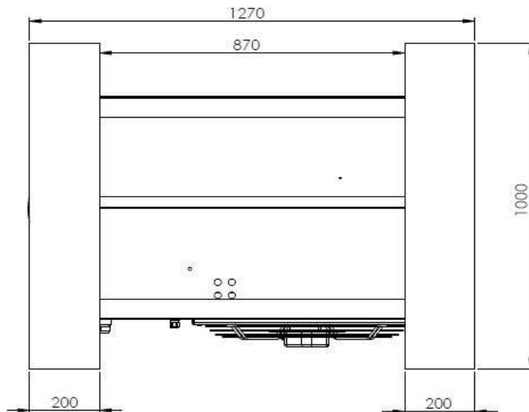
Abb.: Fundamentplan
