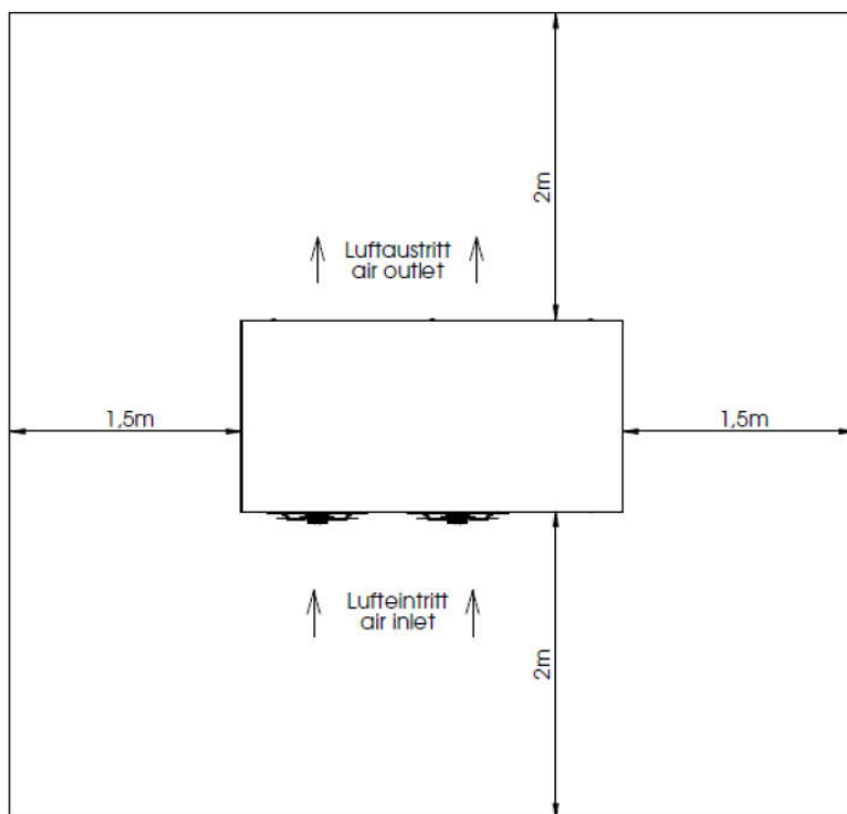
Abb.: Empfehlung der Mindestabstände zu umliegenden Gegenständen bei Aufstellung
