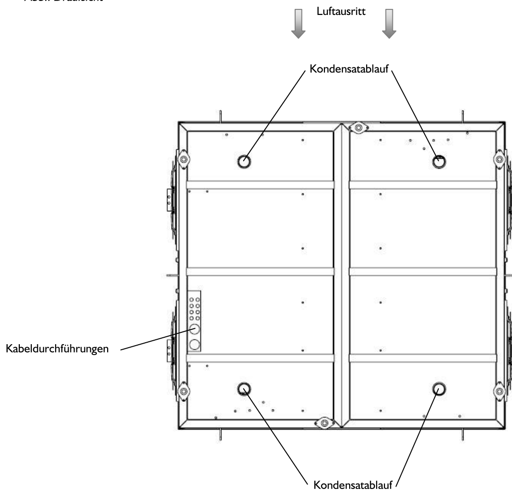
Abb.: Untersicht
