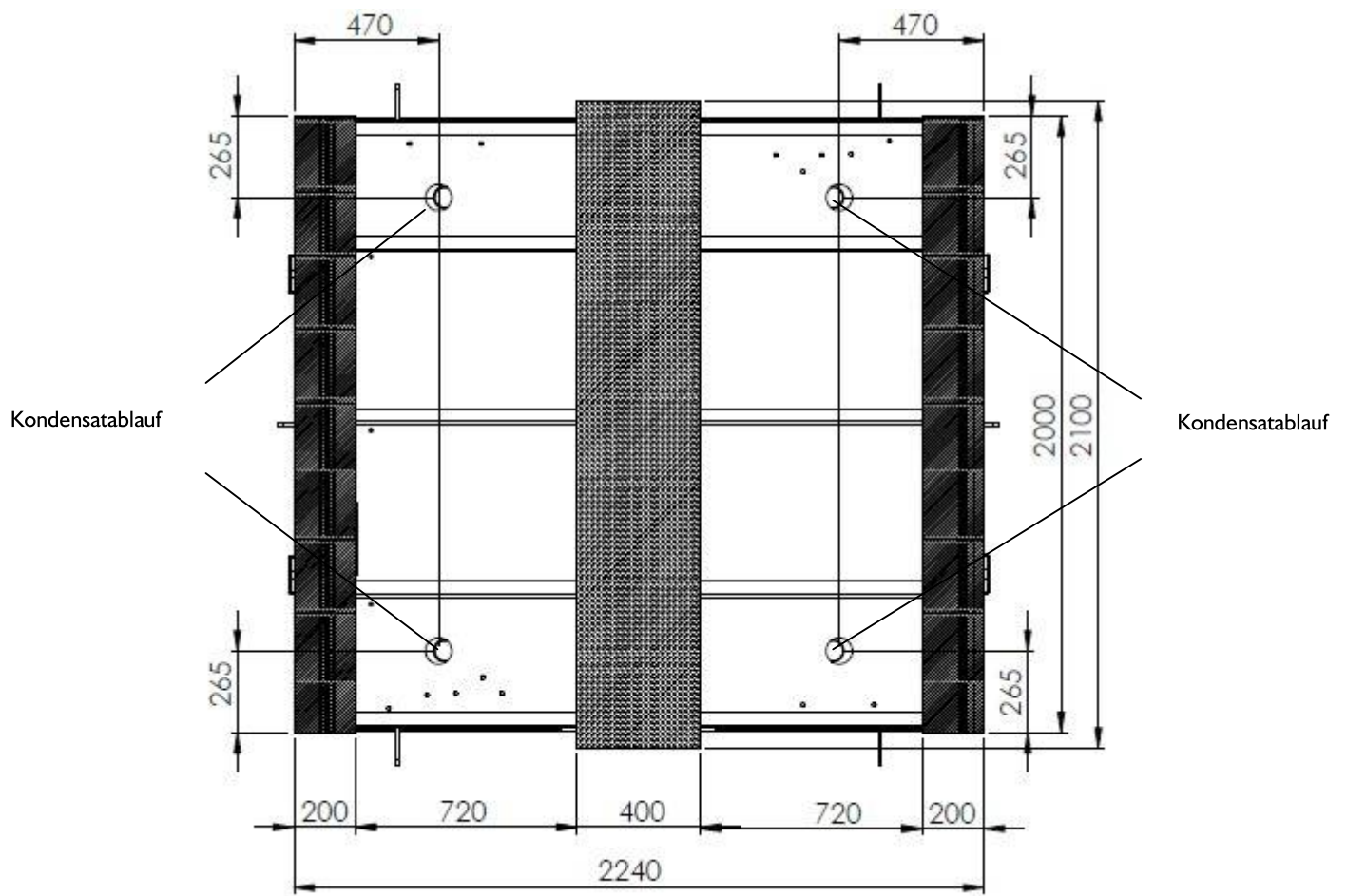
Abb.: Fundamentplan
