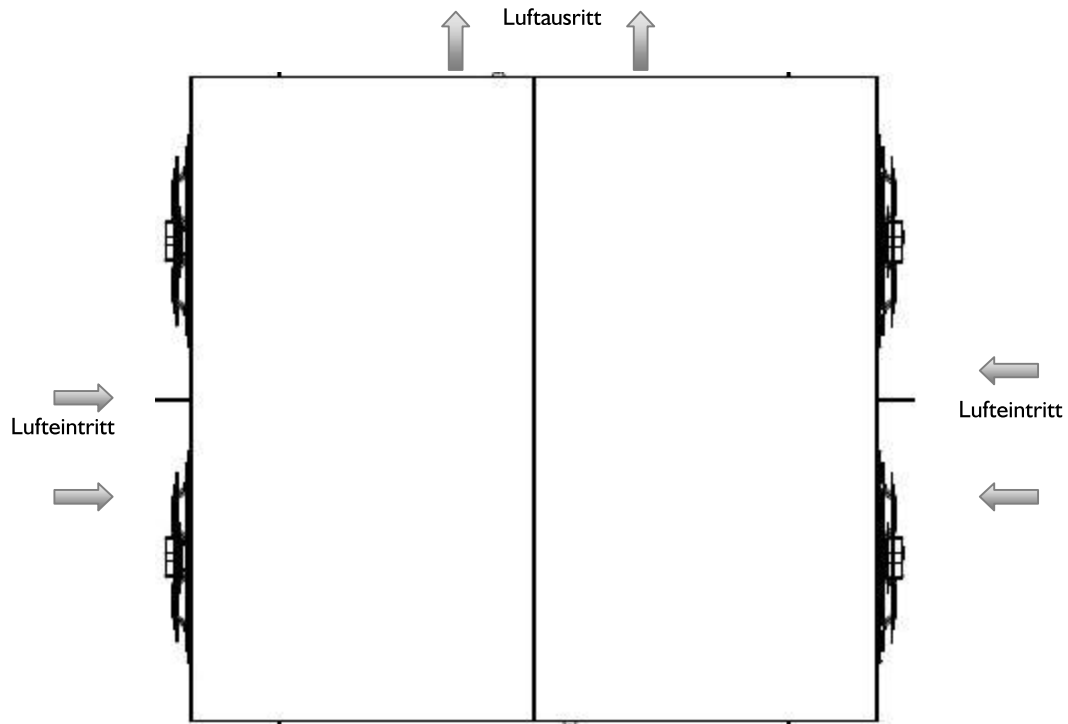
Abb.: Draufsicht
