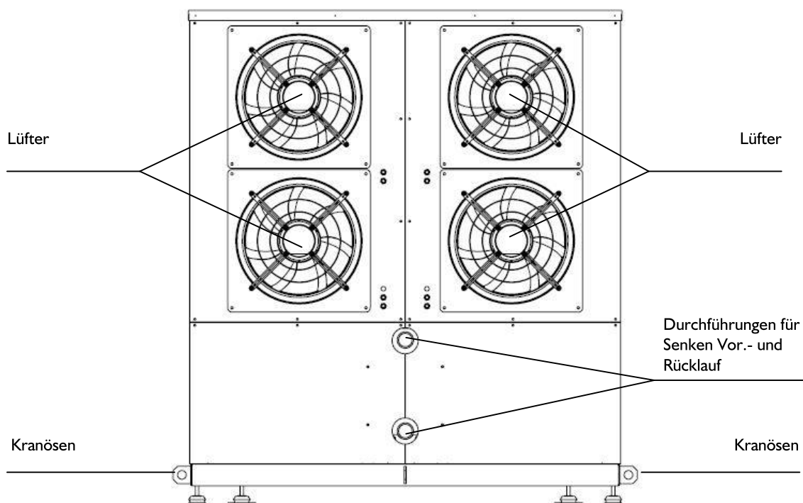
Abb.: Rückansicht
